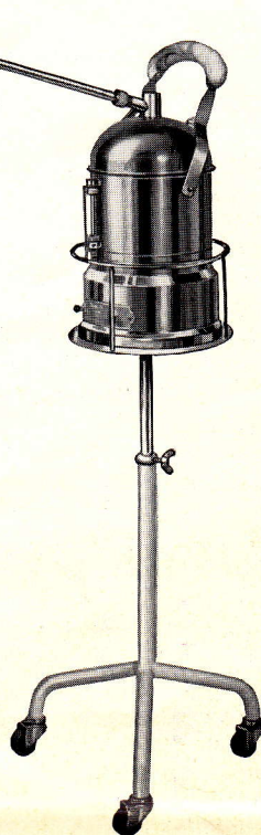
Fahrbarer Ständer Nr. 20 für Geräte der Reihe Nr. 18 / 18a, elfenbein, einbrennlackiert, Ständersteller und Haltegitter Messing hochglanzvernickelt, mit Höheneinstellung und schwenkbaren, kugelgelagerten Gummirollen.
