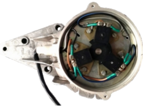
EBZA 2s - Steuerteil mit 3 optoelektronischen Zündgebern
