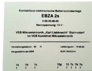
EBZA 2s - Leistungsteil mit 6x SU 177
