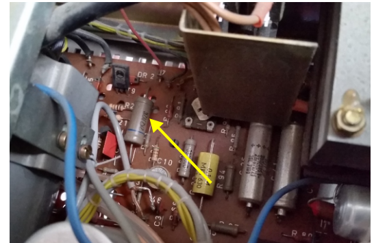
Ausschnitt Leiterkarte EO 211 mit Metallschichtwiderstand
