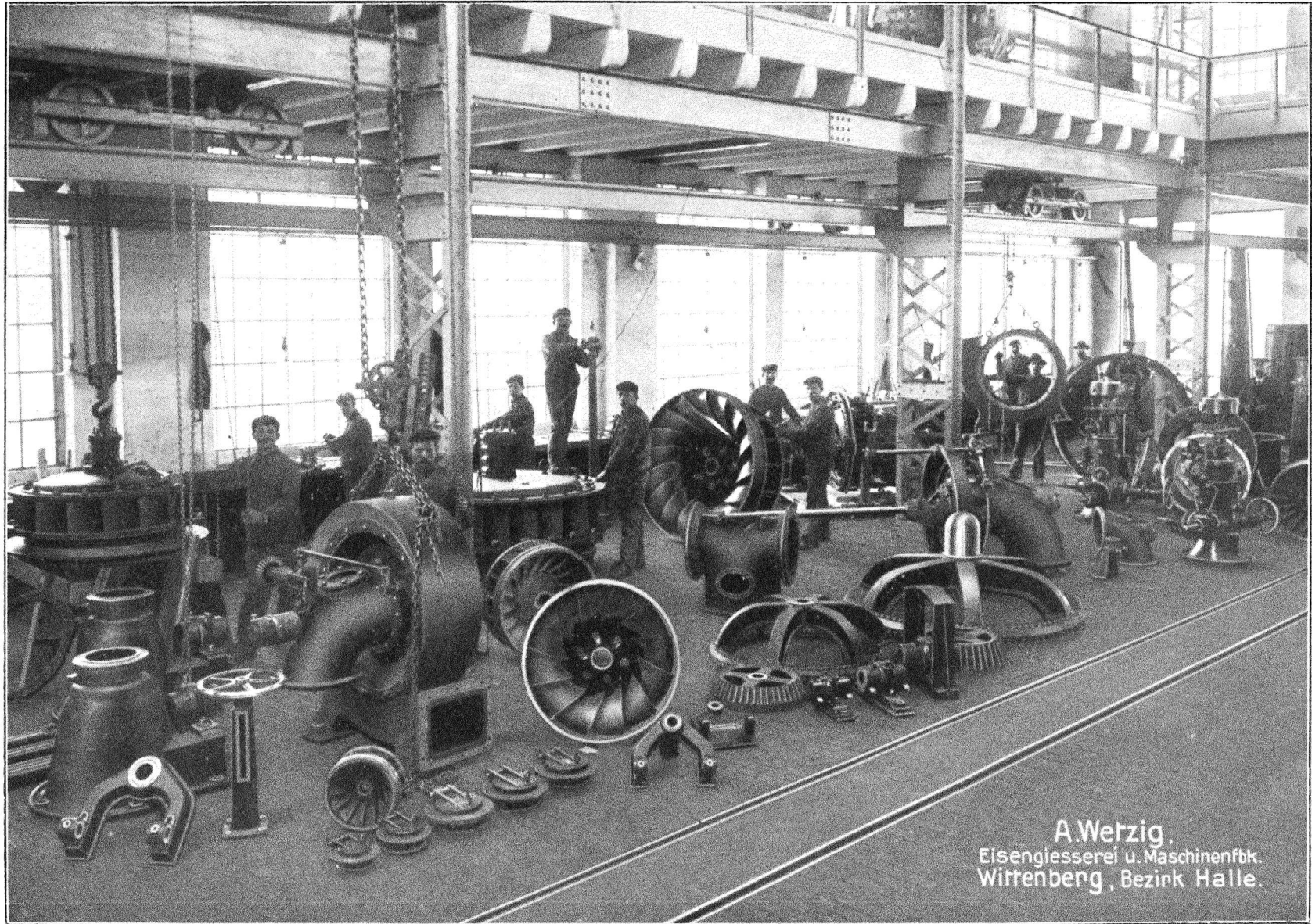
Turbinen-Werkstatt
